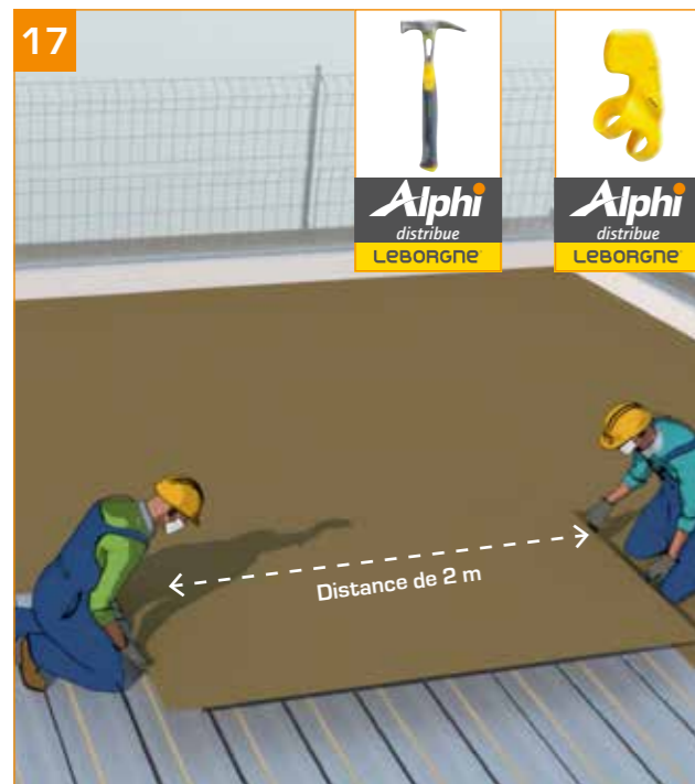
17 - Quand la structure est terminée et réglée en hauteur : mise en place du contre-plaqué (CP). → Sécurité périphérique (voile, poutre...) réalisée au préalable. → Utilisation de la servante pour découpe du contre-plaqué.
