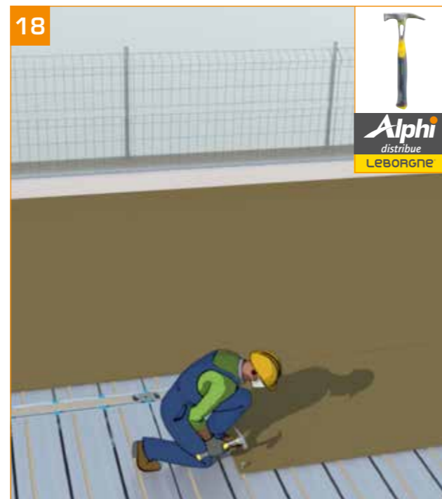
18 - Clouer avec des pointes. - S'assurer de la présence d'un porteur sous le joint des feuilles de CP. - S'assurer de l'étanchéité du coffrage entre feuilles de CP et à la périphérie. Interdiction de circuler sur les panneaux de contre-plaqué, sauf pour le personnel formé et habilité à poser les panneaux de contre-plaqué.
